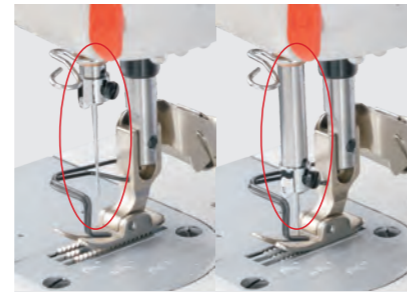
上下停针，自由调节 Needle position, easy to adjust
